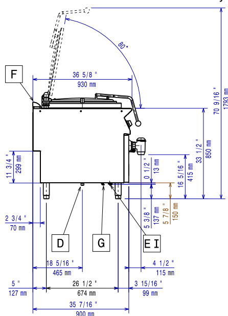
Zij aanzicht
